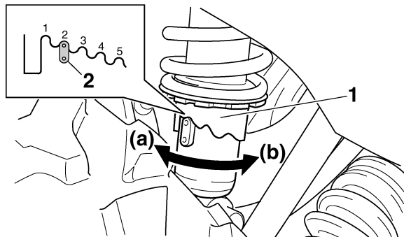
1. Clé spéciale
