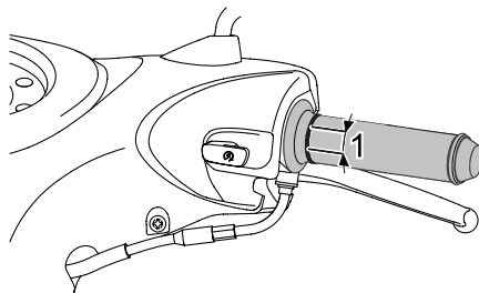
1. Jeu de câble des gaz
