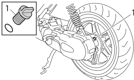
1. Bouchon de remplissage de l'huile de transmission finale
