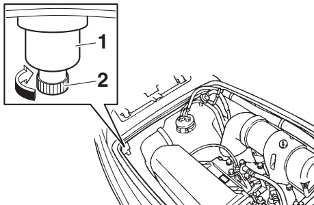
1 Séparateur d'eau
