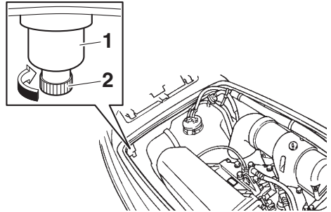
1 Séparateur d'eau
