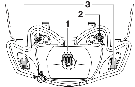
1. Connecteur de phare 2. Fiche rapide de veilleuse 3. Fiche rapide de fil de clignotant
