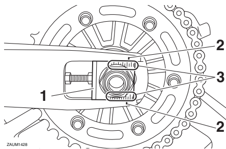
1. Tendeur de chaîne de transmission 2. Encoche 3. Repères d'alignement
