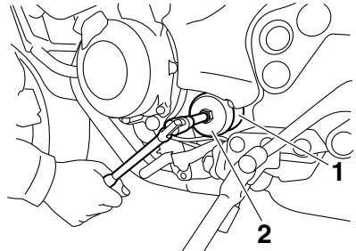
1. Cartouche de filtre à huile 2. Clé pour filtre à huile
