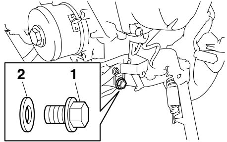
1. Vis de vidange d'huile moteur 2. Joint
