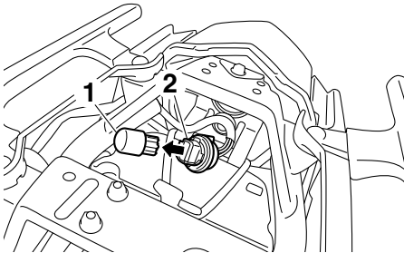
1. Ampoule de feu stop/arrière 2. Douille d'ampoule de feu stop/arrière
