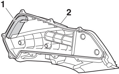
1. Élément de filtre à air secondaire 2. Couverture du boîtier de filtre à air
