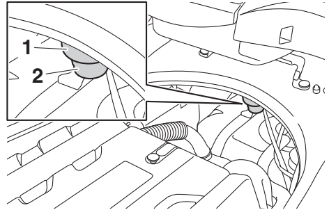
1 Séparateur d'eau 2 Vis de vidange
