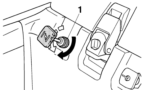
1 Ecrou de réglage du bouton de starter
