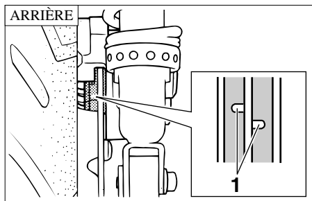
1. Rainure d'indicateur d'usure (×2)
