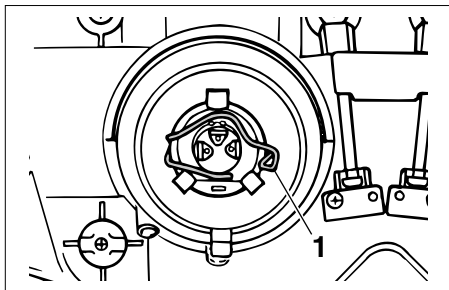
1. Porte-ampoule du phare (×2)
