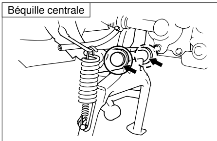
Béquille centrale
