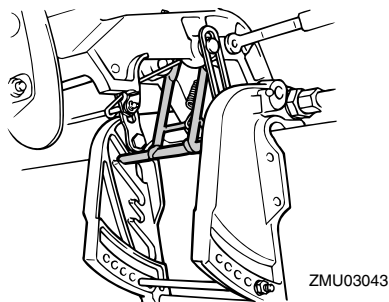
1. Levier(s) de verrouillage du capot
