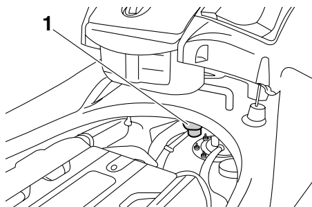
1 Séparateur d'eau
