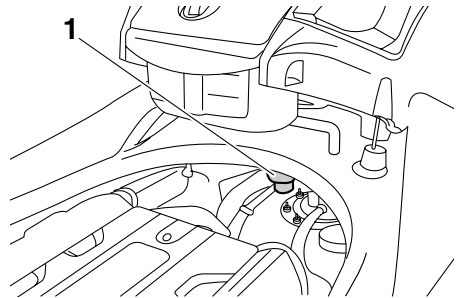
1 Séparateur d'eau
