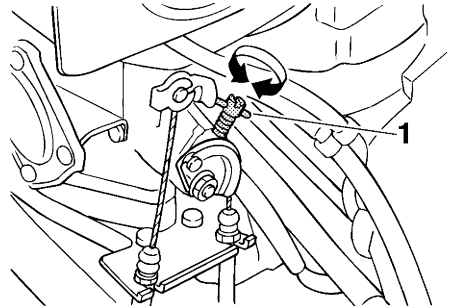
1 Vis de butée de papillon
