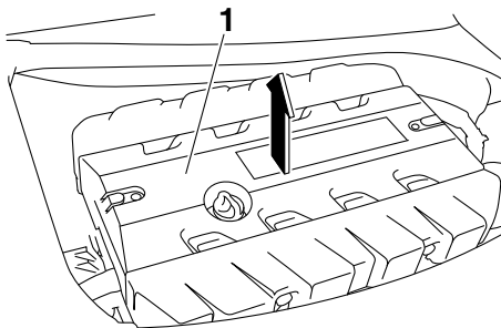
1 Cache du moteur
